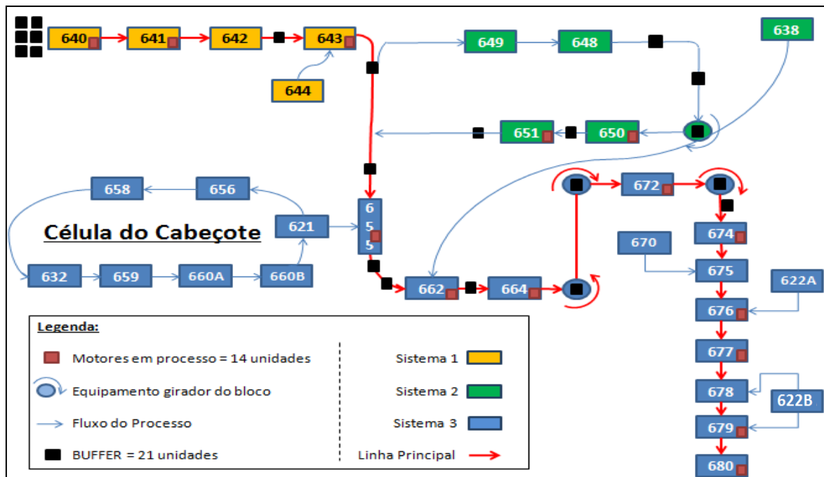
FIGURA 4 - LAYOUT DA LINHA FONTE: OS AUTORES
