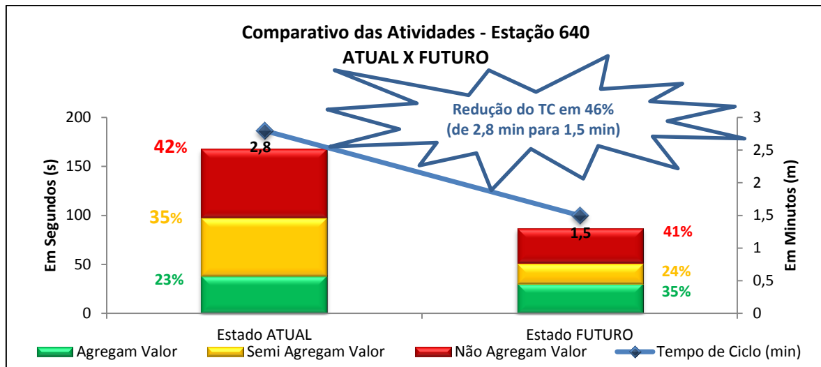
FIGURA 6 - COMPARATIVO DAS ATIVIDADES ATUAL E FUTURO NA ESTAÇÃO 640 FONTE: OS AUTORES
