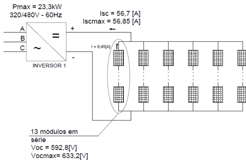
FIGURA 2: DISPOSIÇÃO DAS PLACAS SOLARES FONTE: AUTORES (2018)
