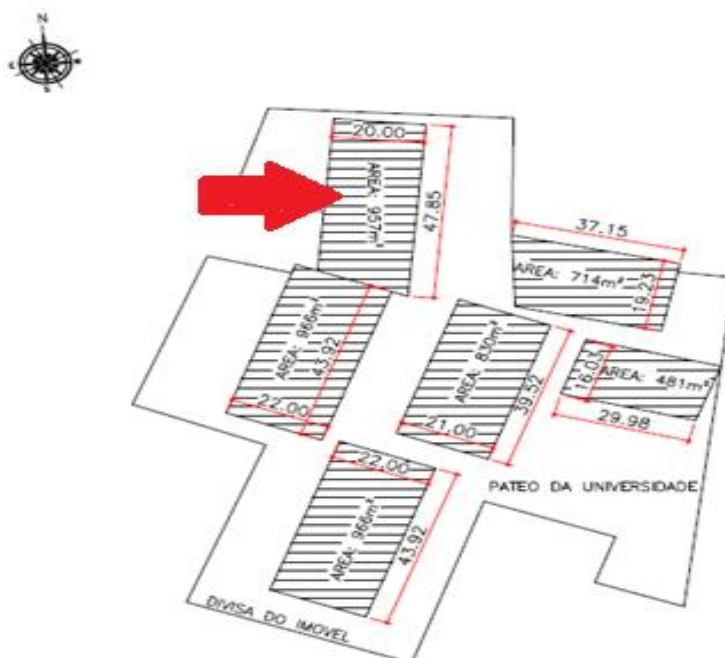
FIGURA 1: PLANTA DA UNIFACEAR CAMPUS ARAUCÁRIA FONTE: UNIFACEAR (2018)
