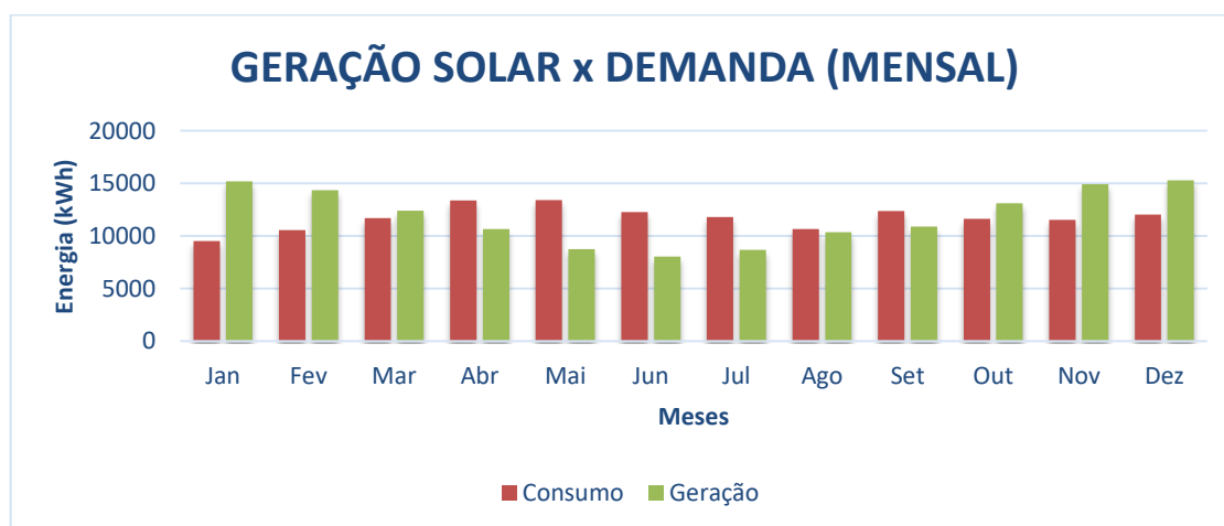
GRÁFICO 1: GERAÇÃO SOLAR X DEMANDA (MENSAL)
