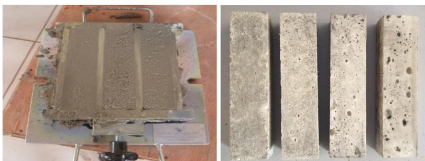
FIGURA 8: CP'S PRISMATICOS. FONTE: AUTORES (2018)
