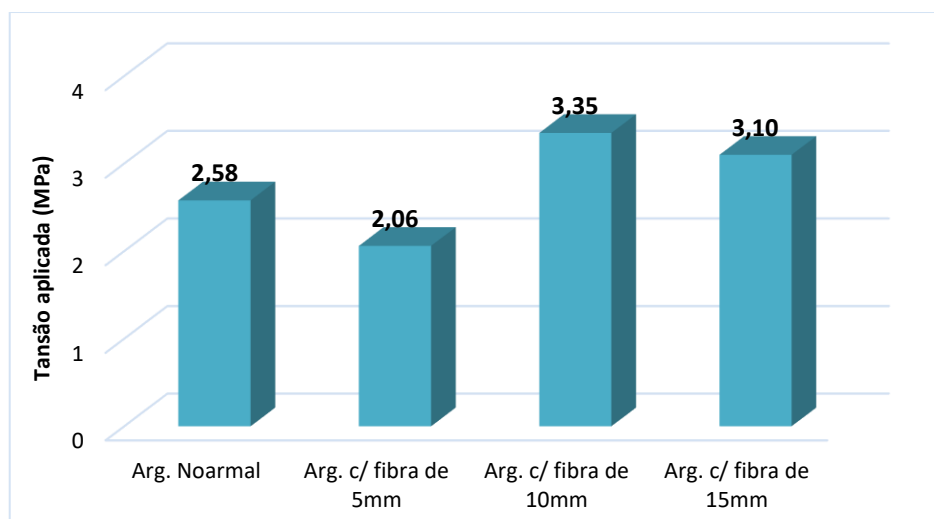
FIGURA 12: RESISTÊNCIA MÉDIA A TRAÇÃO NA FLEXÃO DOS TRAÇOS.
