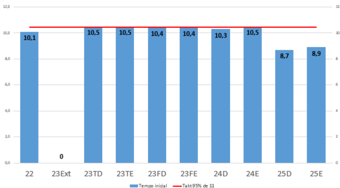
FIGURA 4: SITUAÇÃO ATUAL: TEMPOS PARA CADA POSTO DE TRABALHO FONTE: AUTORES (2018)
