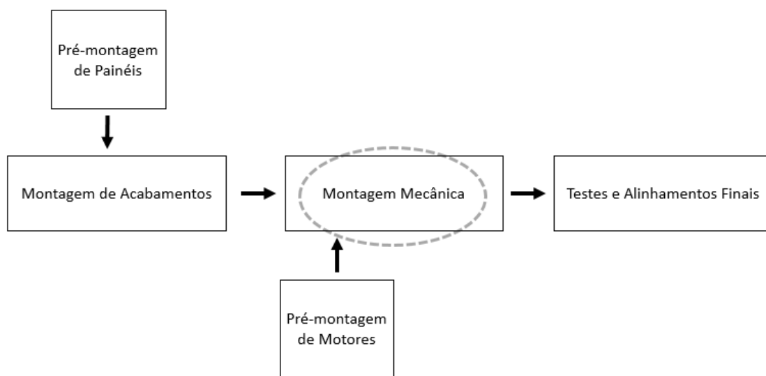
FIGURA 1: FLUXOGRAMA DO PROCESSO FONTE: AUTORES (2018)
