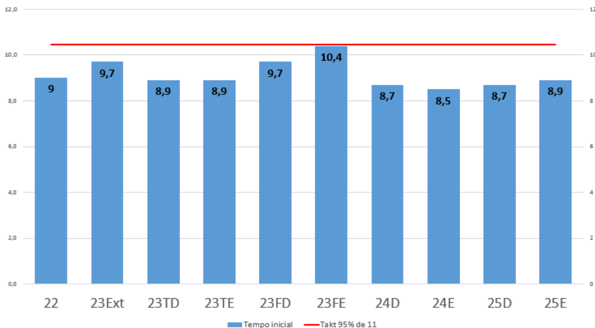
FIGURA 3: SITUAÇÃO INICIAL: TEMPOS PARA CADA POSTO DE TRABALHO FONTE: AUTORES (2018)
