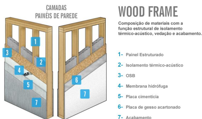
FIGURA 1: CAMADAS DO PAINEL DE WOOD FRAME (PAREDE) FONTE: TECVERDE (2015)
